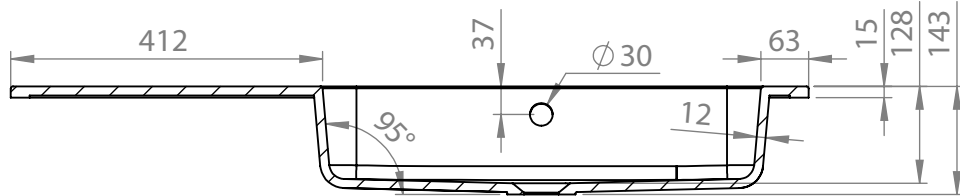
PRZEKRÓJ M-M
